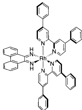
\Delta -[Rh(DPB) 2 phi] 3+ (66)
